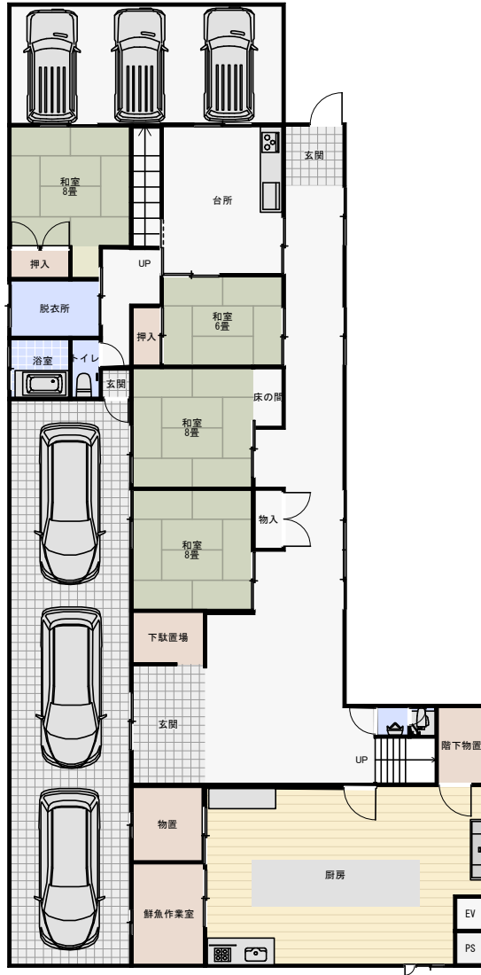
2階 縮尺 1/200
