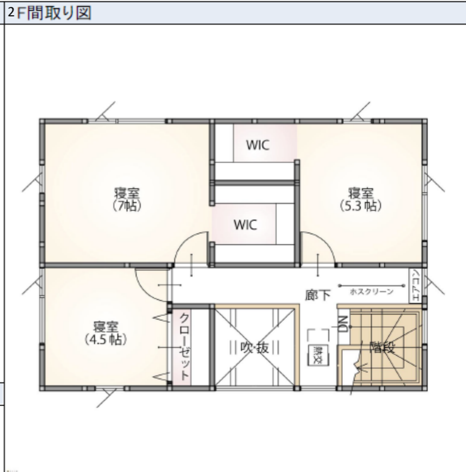
2F間取り図
